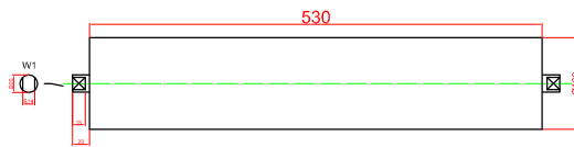
Krażnik nośny gładki \text{Ø}108 \times 530 \times 20 \times 15 \times \text{S}14 PT200
