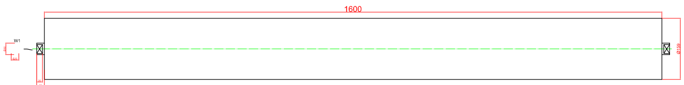
Krażnik odciskowy gładki \text{Ø}159 \times 1600 \times 25 \times 20 \times \text{S}20 PT200
