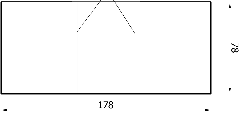
Rozwinięcie blachy poz.1
