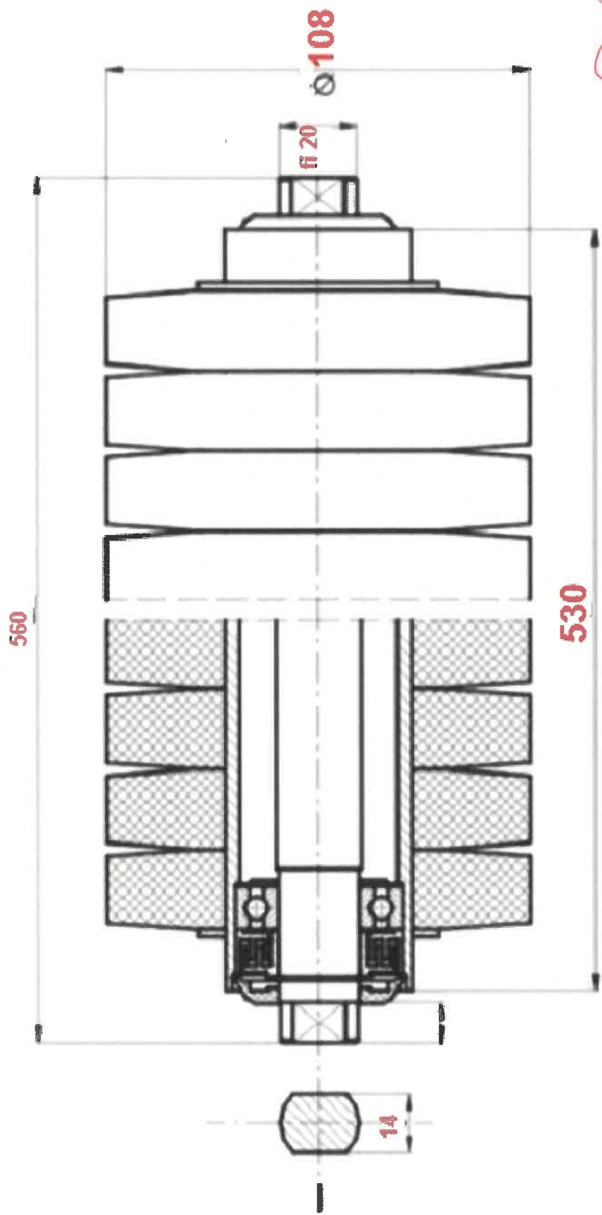
Przenośnik P-200 - Krążnik pierścieniowy \varnothing 108 \times 530 \times 20 \times 15 (indeks: 110027416)
