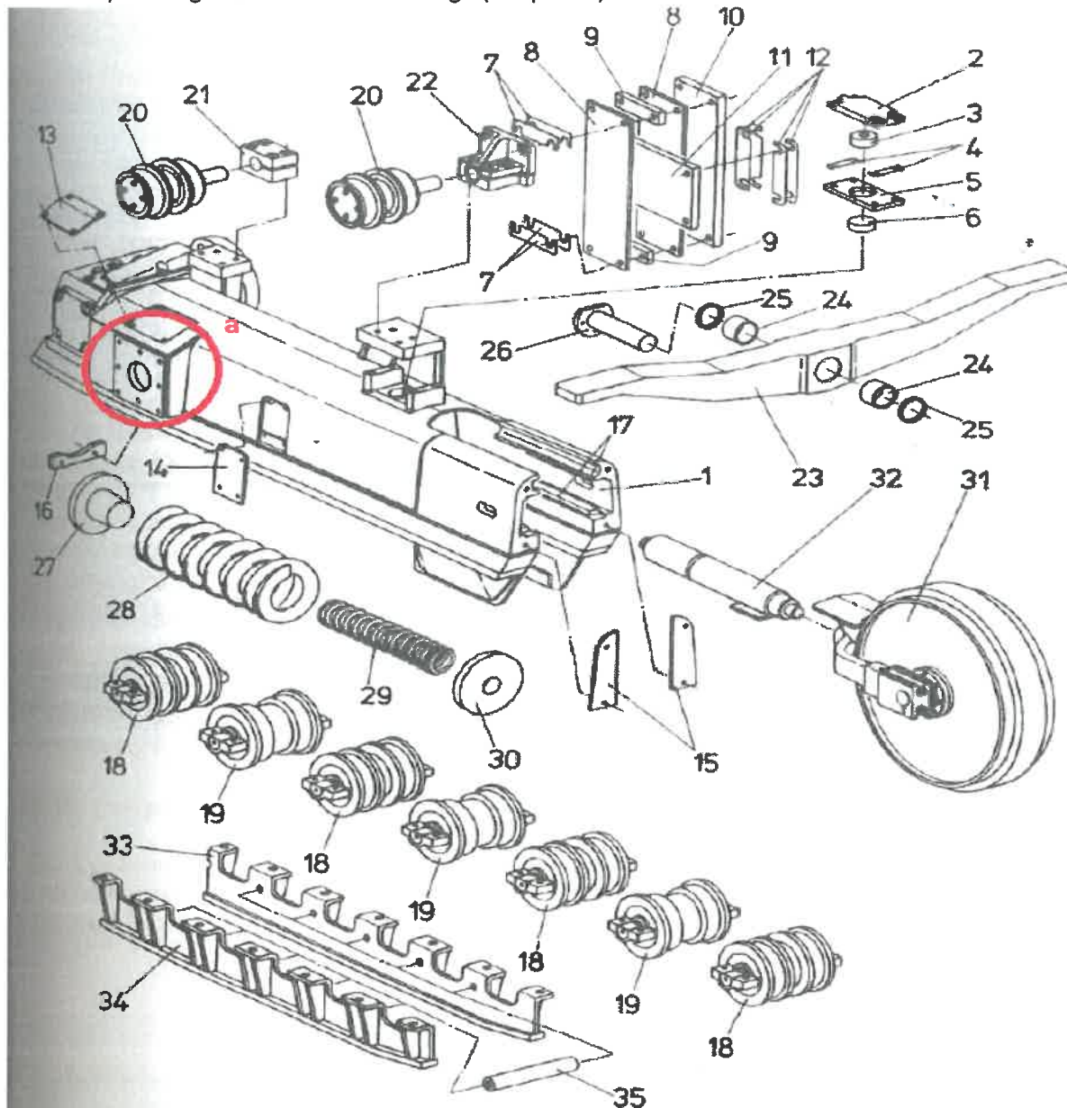
Rys.1 poglądowy podwozia.
