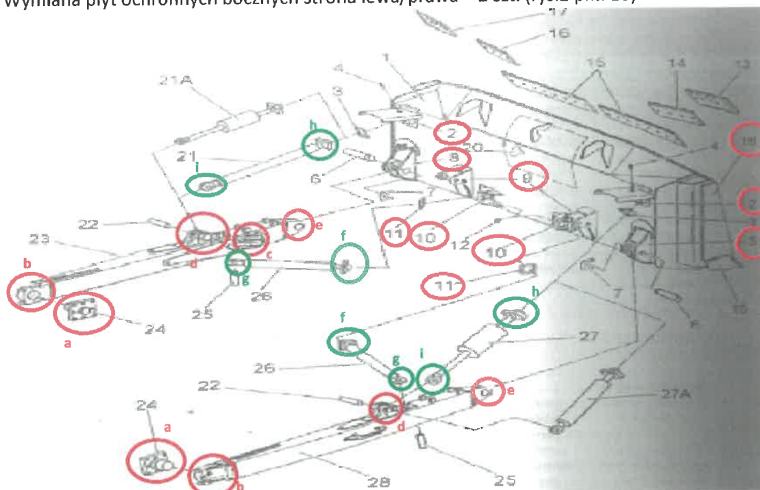
Rys. 2 poglądowy mocowania lemiesza.
