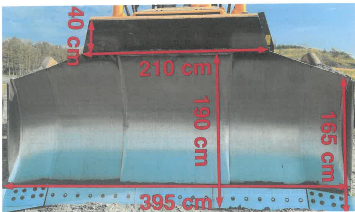
Rys.3 poglądowy poszycia lemiesza.
